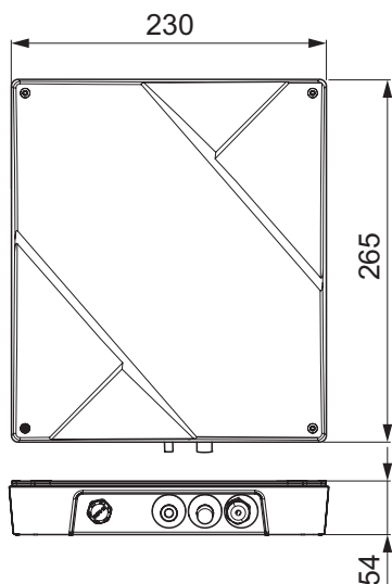
Staub- und wasserdichtes IP65-Kit
